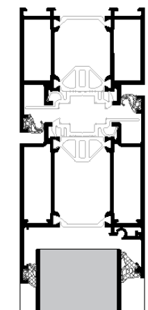
Nebeneingangstüre 4 U_D – Wert ab 1,2 w/m^2k Glaslichte = 150x1530mm
